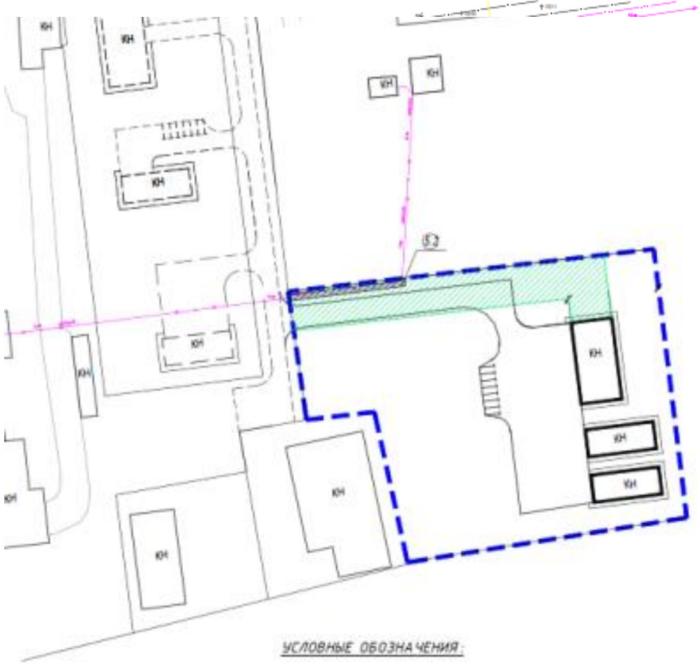
СХЕМА ИНЖЕНЕРНО-ТЕХНИЧЕСКОГО ОБЕСПЕЧЕНИЯ ЗЕМЕЛЬНОГО УЧАСТКА М 1:1000
